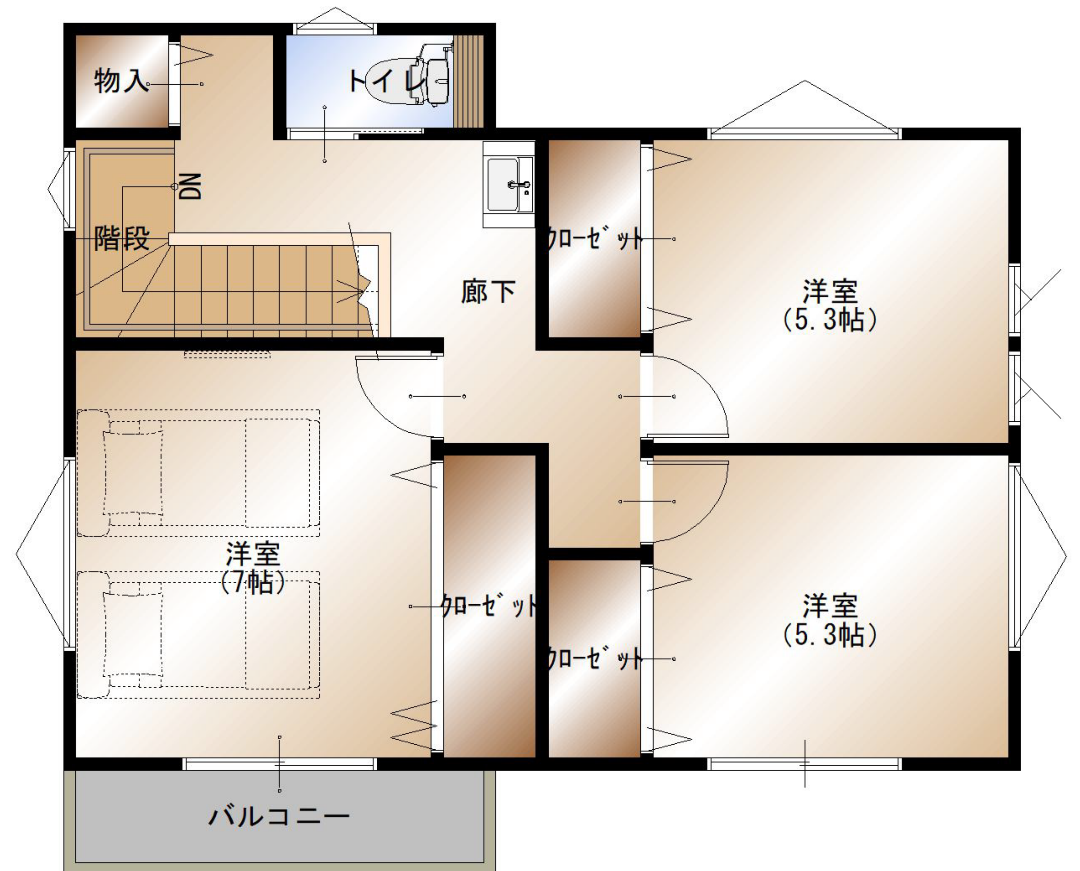
2 階
